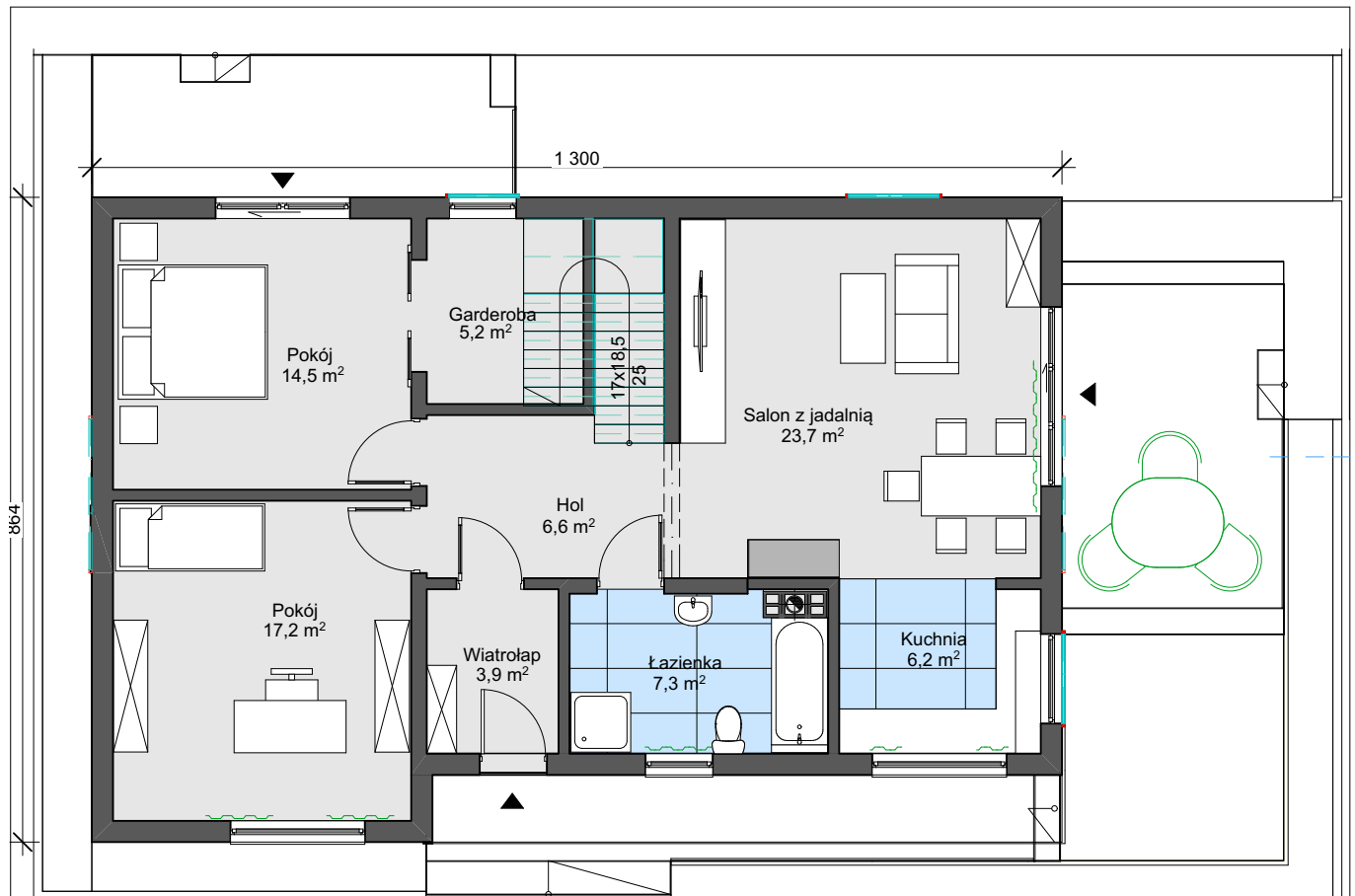
RZUT PRZYZIEMIA SKALA 1:100
