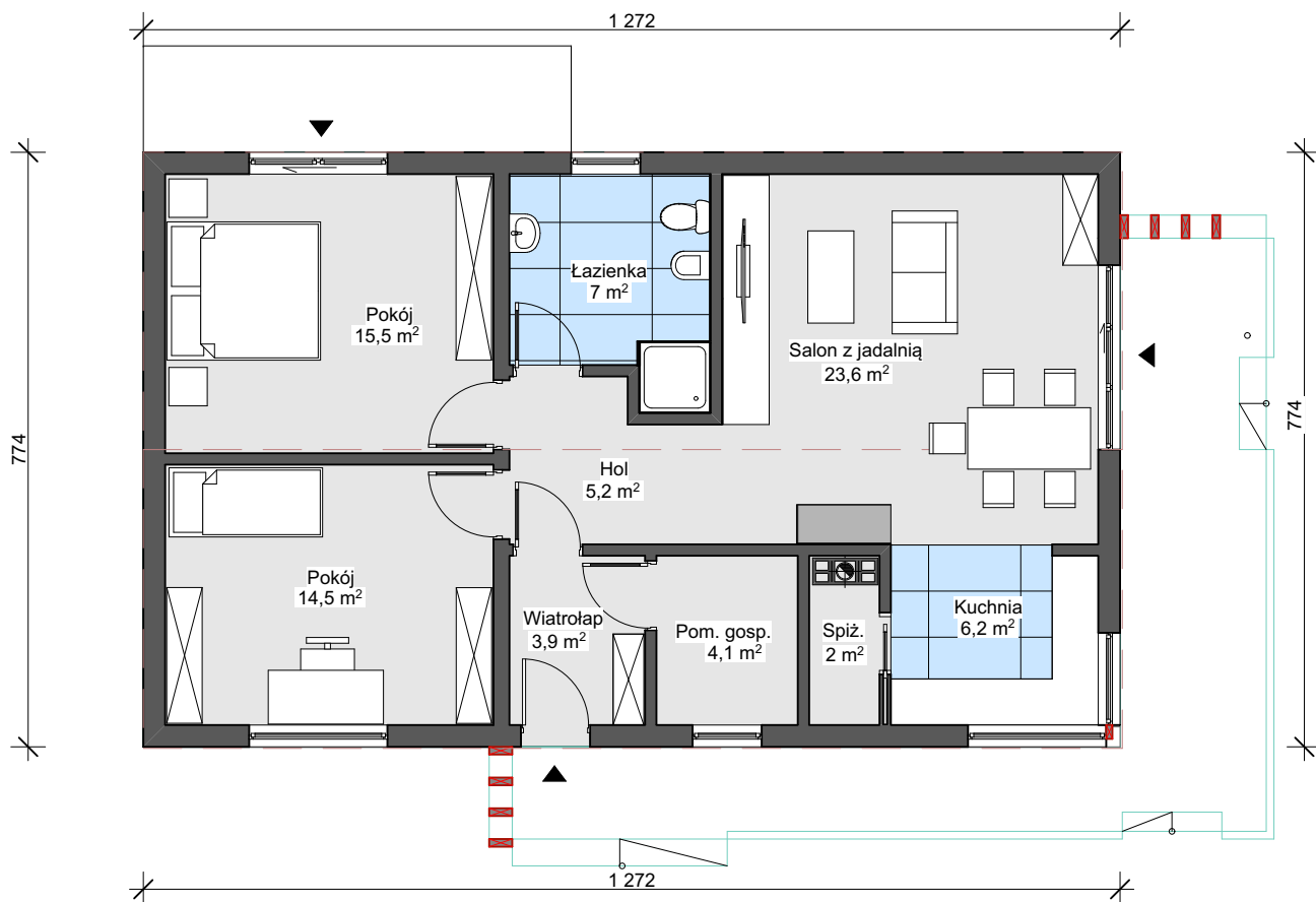
RZUT PRZYZIEMIA WARIANT 1 SKALA 1:100
